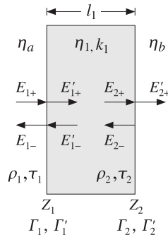
Fig. 5.4.1 Single dielectric slab.
