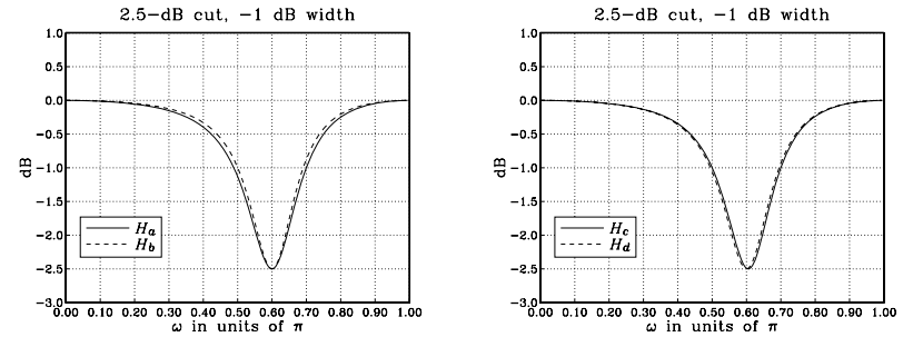
Fig. 11.4.3 Parametric EQ filters.
