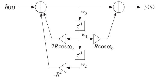
Fig. 8.1.2 Digital cosinusoidal generator
