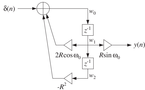
Fig. 8.1.1 Digital sinusoidal generator
