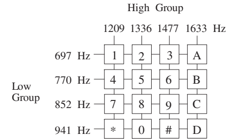
Fig. 8.1.3 DTMF keypad.
